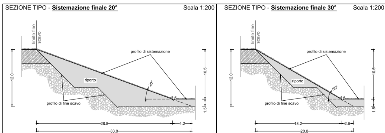
Figura 14: schema di rivestimento delle scarpate di fine scavo definitive, a sinistra, e provvisorie, a destra; a destra lo schema di rinfiacco di eventuali scarpate provvisorie che si verrebbero a configurare in direzione ovest, sud ed est qualora si rendesse possibile entro i termini dell'autorizzazione ipotizzare lo sfondamento dei setti e/o delle scarpate perimetrali.
