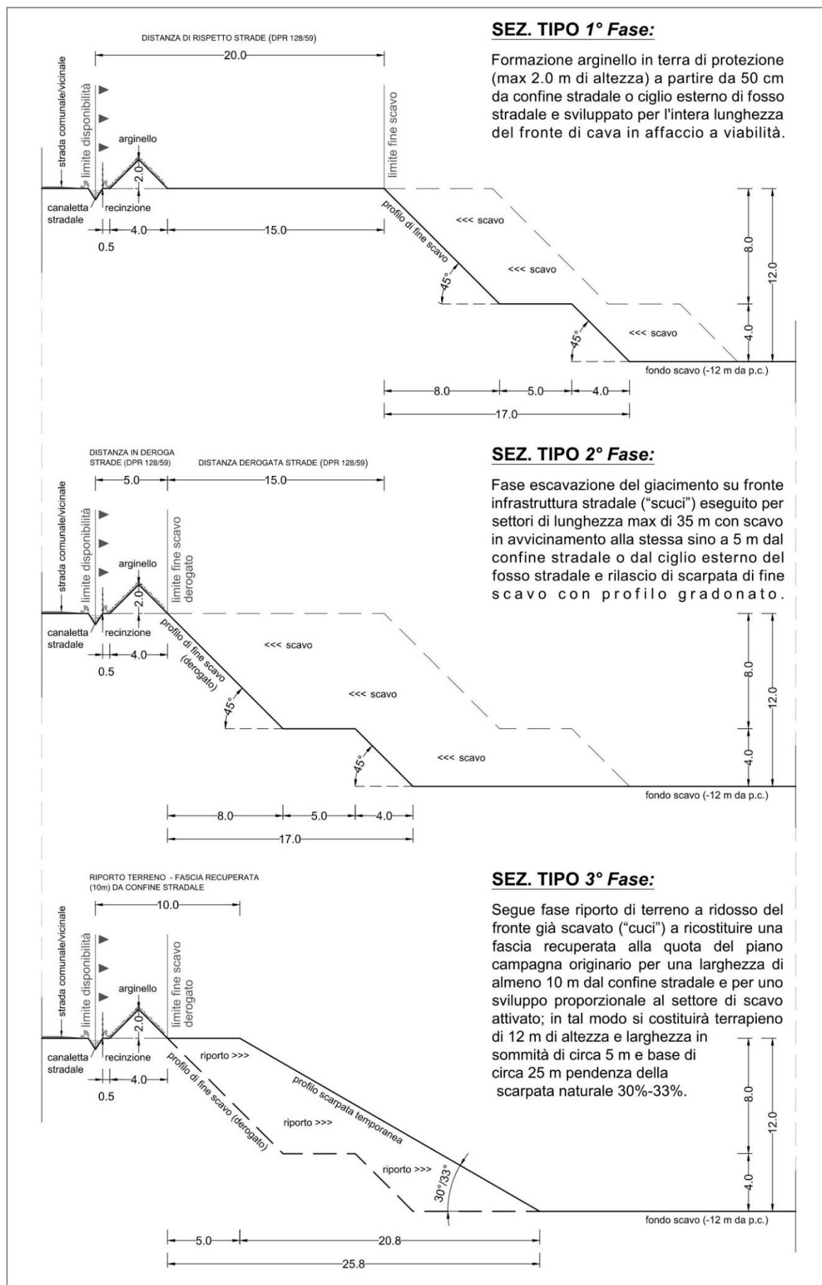
Figura 12: Schema modalità di coltivazione tipo "cuci-scuci" (tratto da PC2024 – "Proposta di coltivazione area di cava in prossimità della viabilità pubblica in deroga alle distanze di cui all'art.104 del D.P.R. 128/59").
