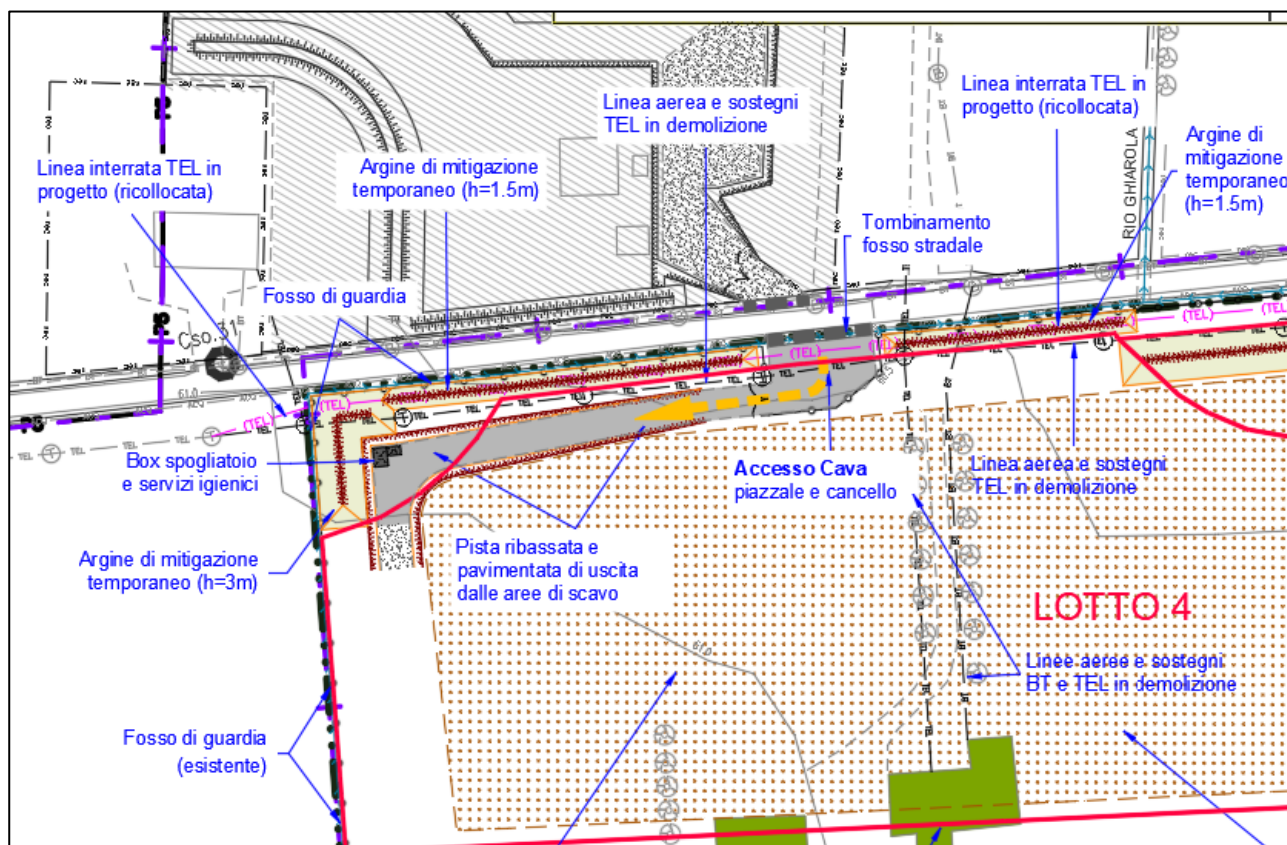
Figura 9: Stralcio di tavola T3 "Opere preliminari"; realizzazione del piazzale di accesso su Strada Pederzona.
