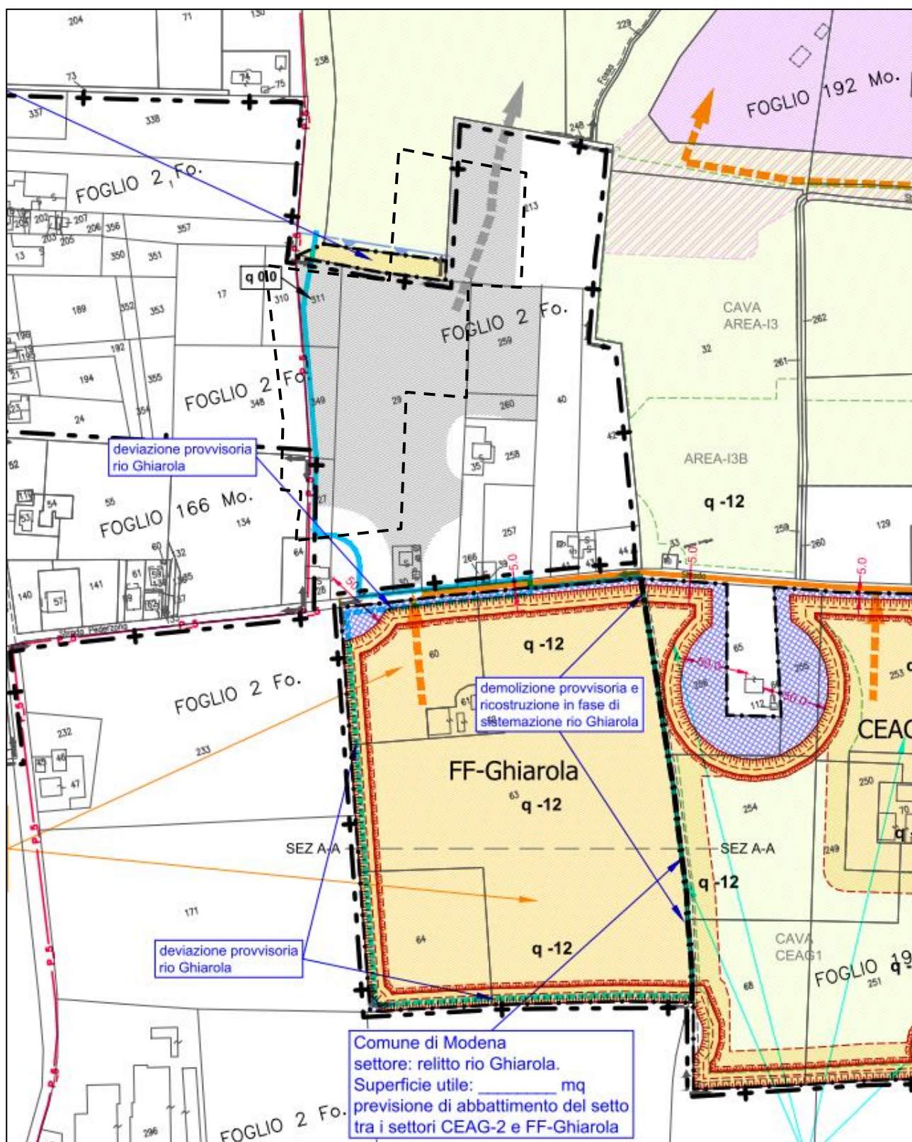
Figura 4: Estratto della tavola 2.2.g del PC2024 "Progetto - Ipotesi di scavo fino alla concorrenza di 1'449'240 mc"; l'area di intervento è perimetrata con tratteggio nero.
