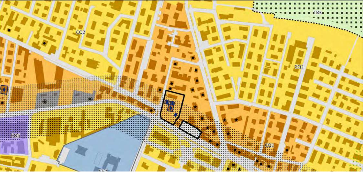
PUG - CARTA DELLA TRASFORMABILITÀ scala 1:5000
