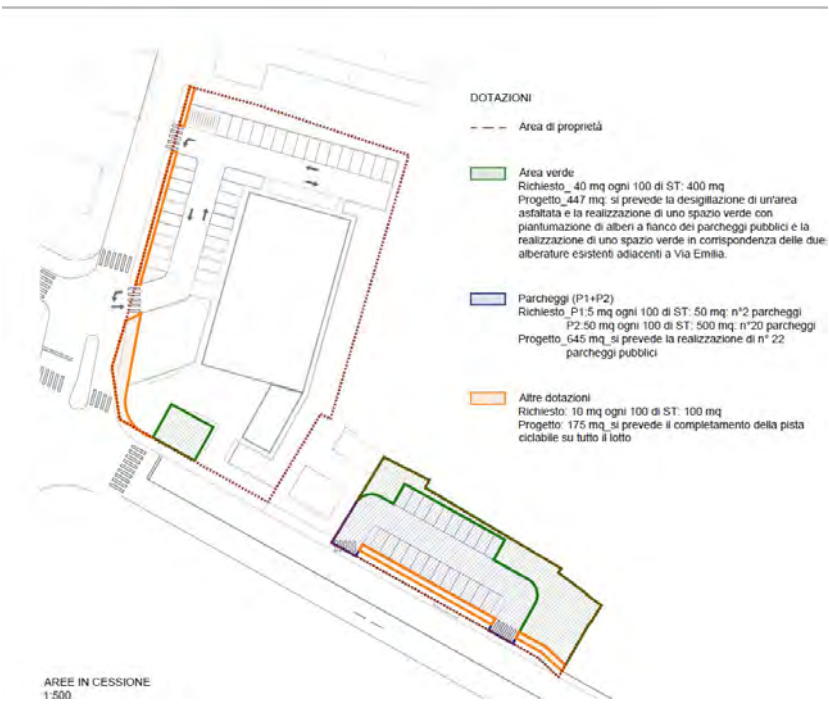
PROGETTO PROPOSTO - AREE DI CESSIONE
