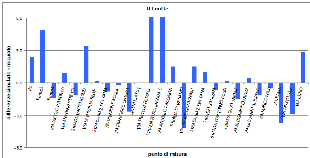
Figura 4: \Delta L_{N_{notte}} tra livello simulato e misurato in ogni punto di misura
