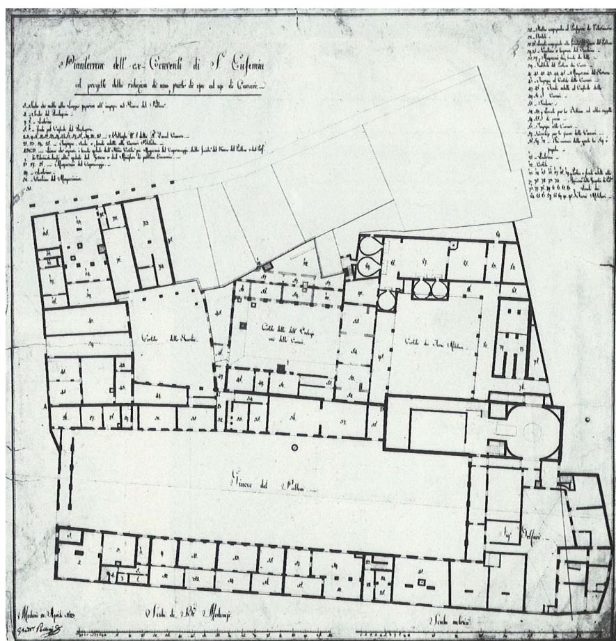
COMPLESSO CONVENTUALE DI S. EUFEMIA – "Pianterreno dell'ex Convento di S. Eufemia, col progetto della riduzione di una parte di esso ad uso di Carcere". Anno 1829. (ASMo, Governatorato, n.2. Inchiostri policromi).
