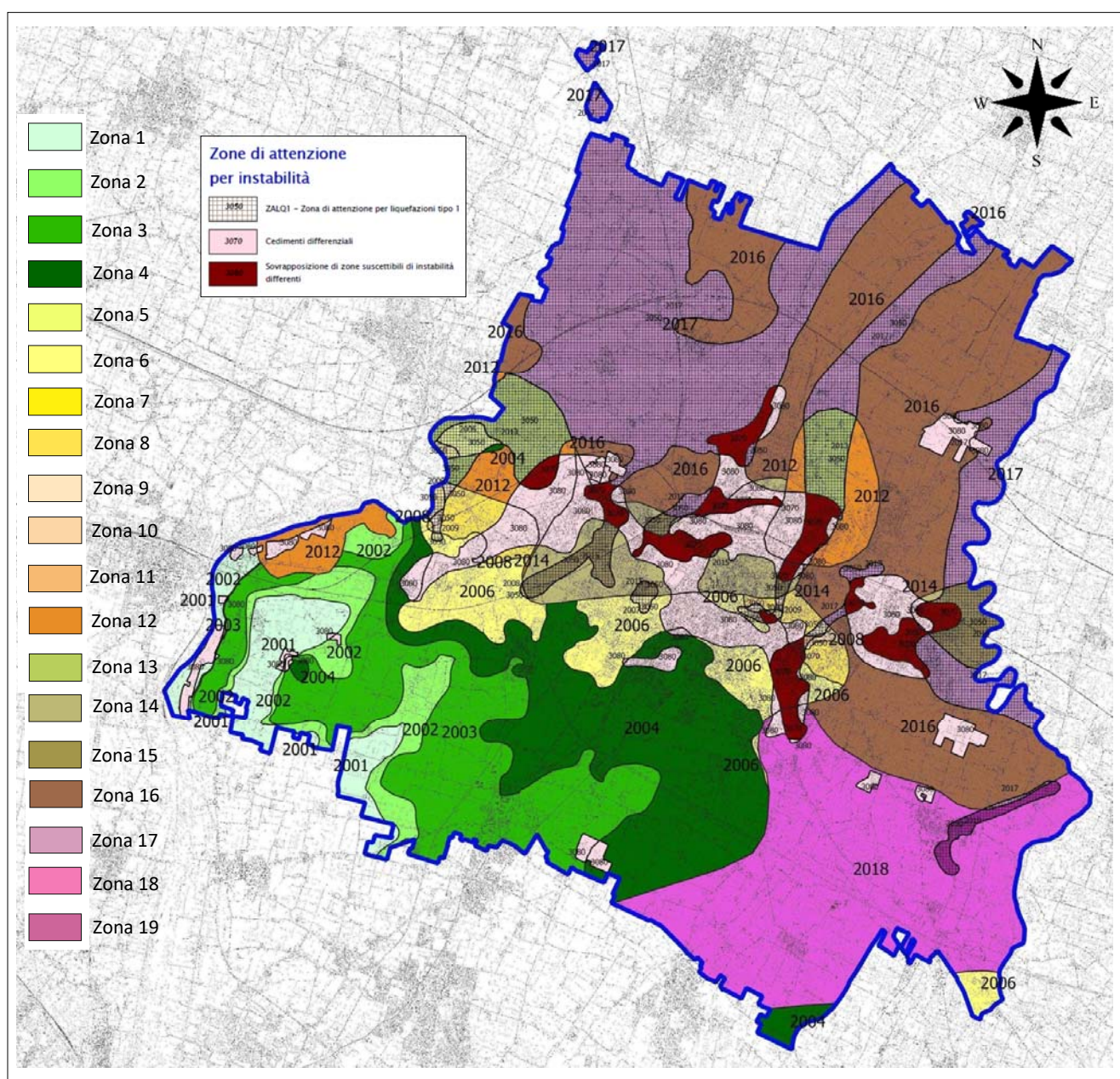
FIGURA 49: CARTA MICROZONE OMOGENEE IN PROSPETTIVA SISMICA (MOPS)
