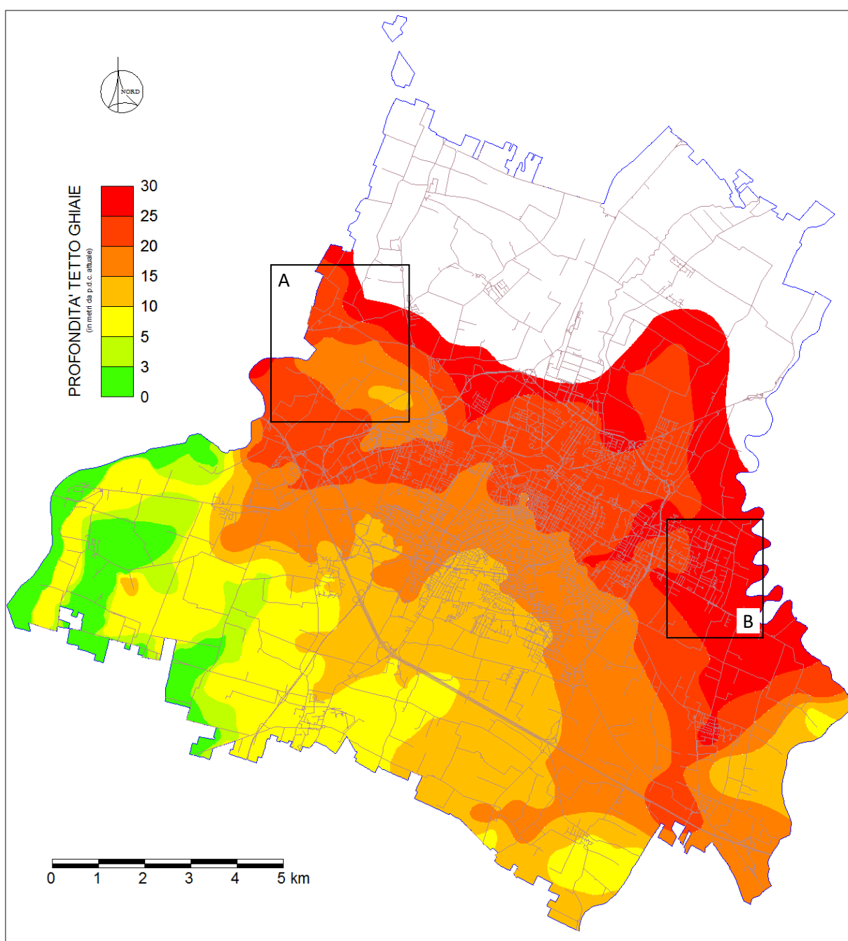
FIGURA 26: CARTOGRAFIA DEL TETTO DEI DEPOSITI GHIAIOSI
