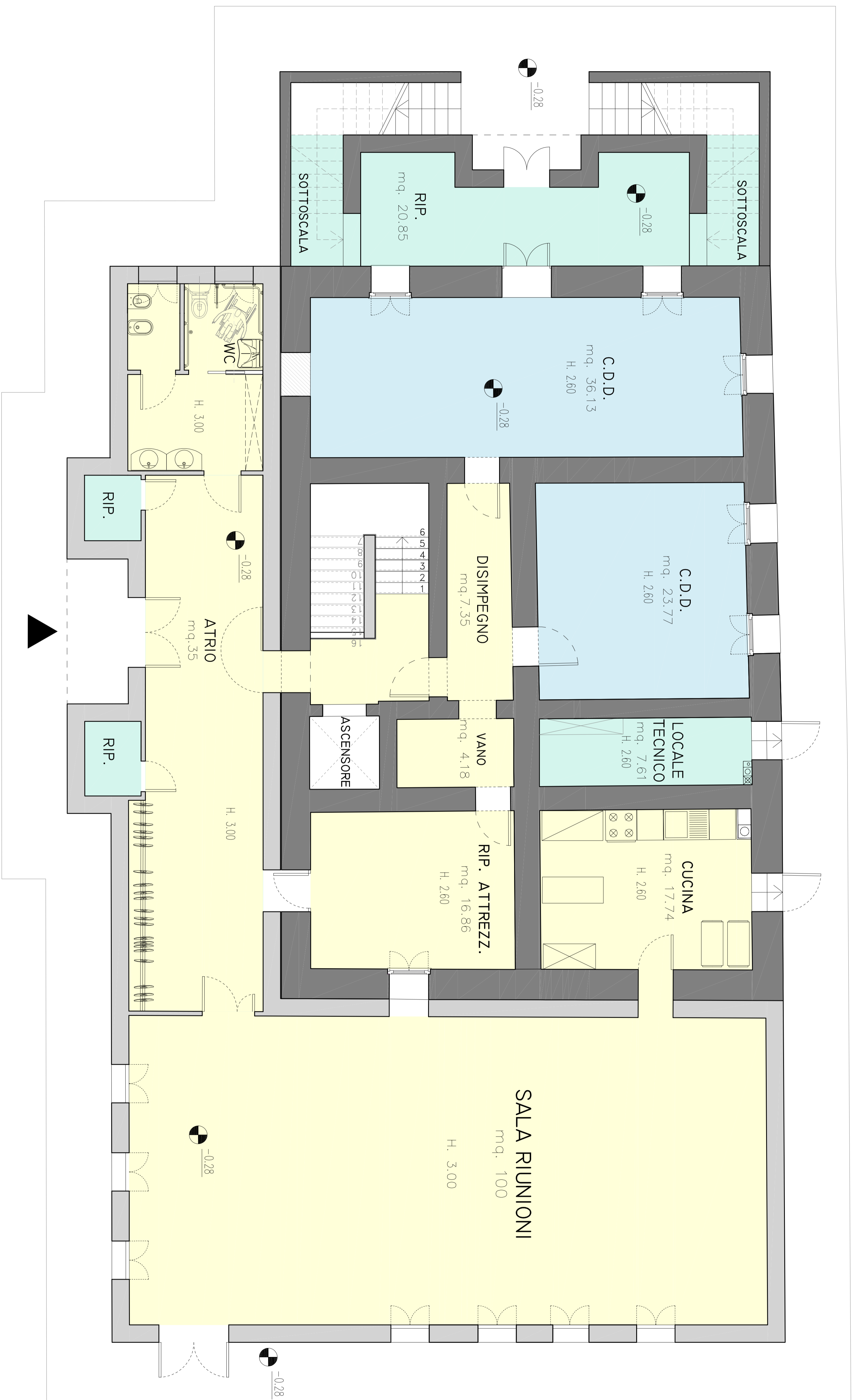
PIANTA PIANO TERRA
